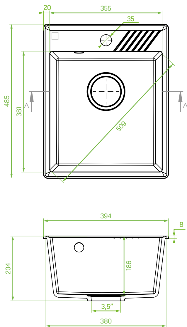
PRZEKRÓJ A-A
